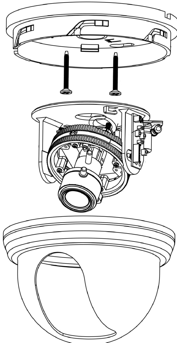
Рис.2.1.1. Установка видеокамеры LTV-CDH-720-V на потолок/стену
