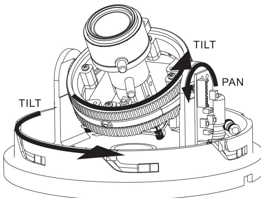
Рис.1.3.1. Настройка положения видеомодуля LTV-CDH-720-V2.8-12
