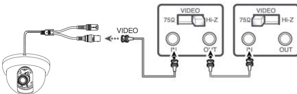
Рис.3.1.2. Подключение видеокамеры LTV-CDH-720-V2.8-12 к монитору
