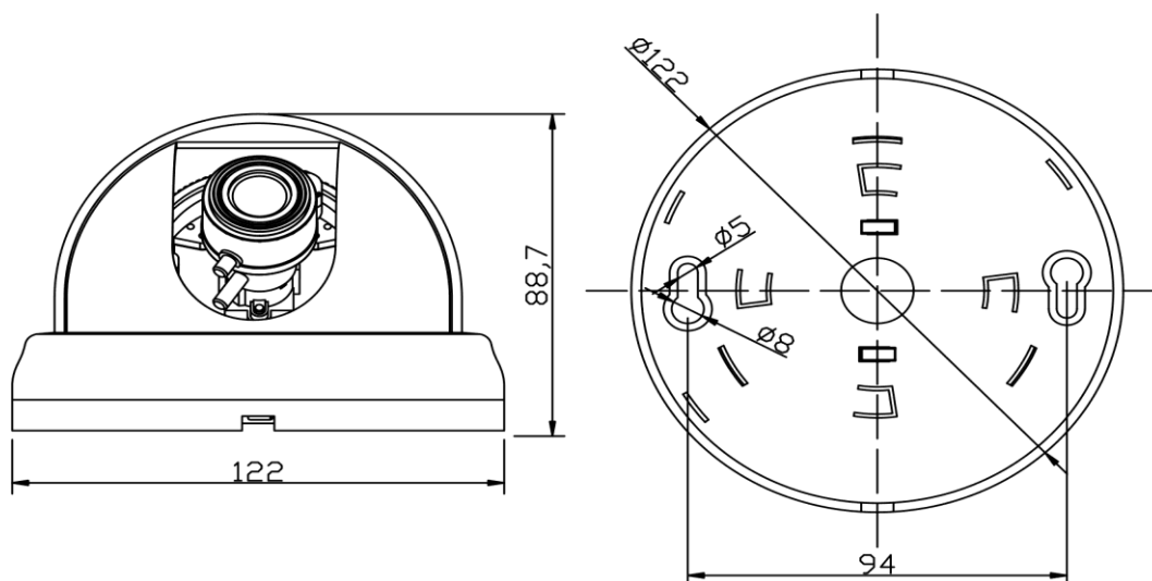
Рис.1.4.1. Габаритные размеры видеокамеры LTV-CDH-720-V2.8-12
