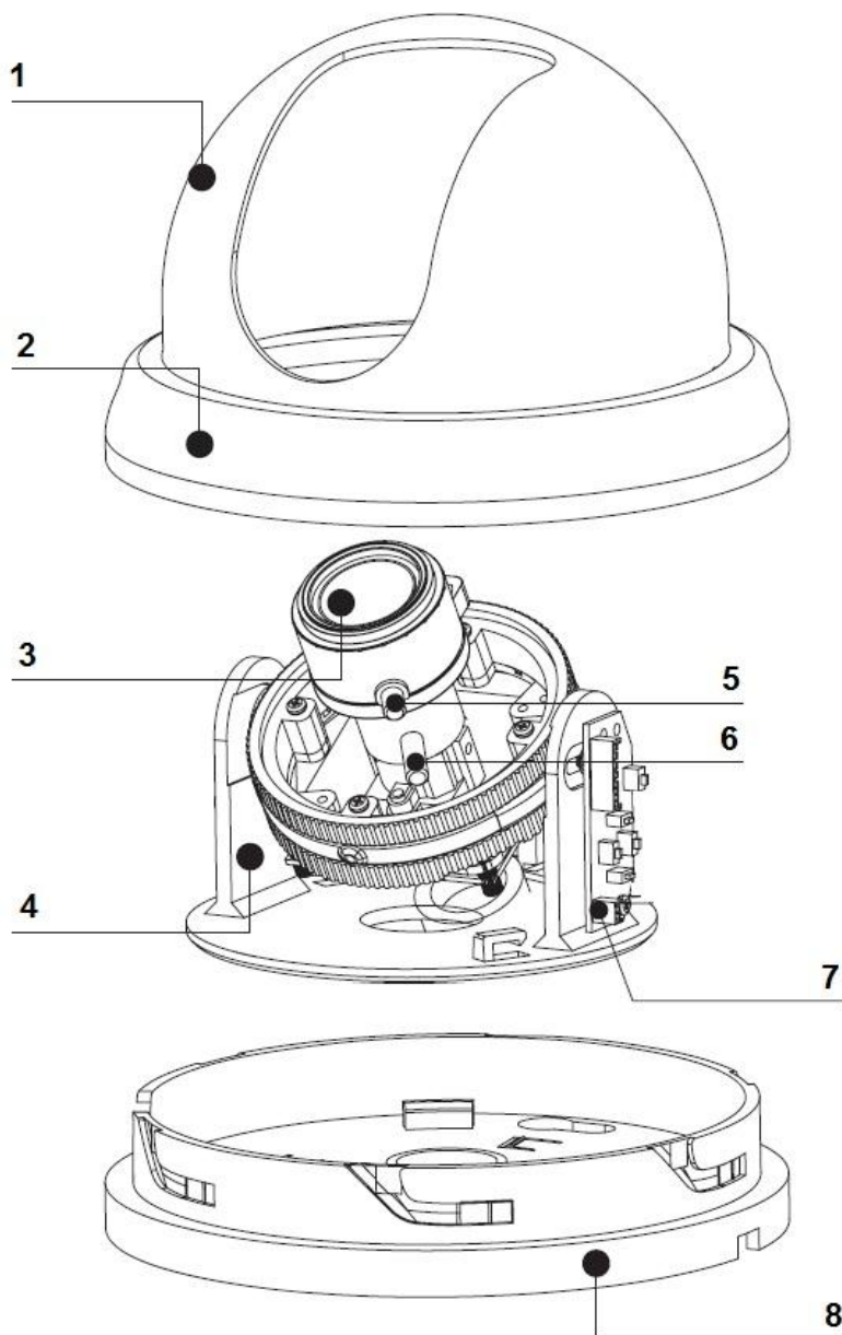
Рис.1.2.1. Основные компоненты видеокамеры LTV-CDH-720-V2.8-12
