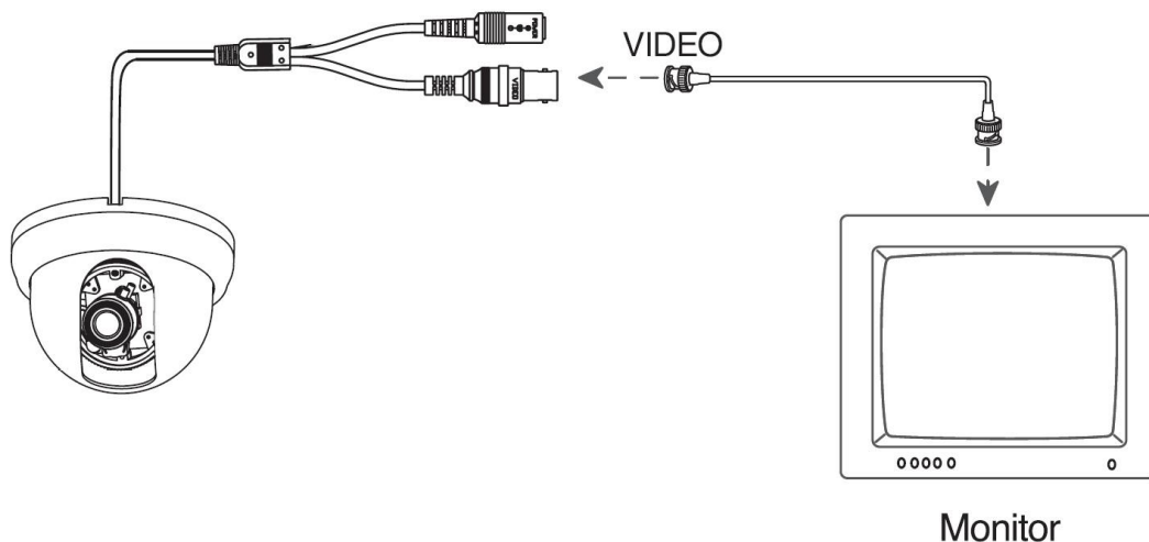
Рис.3.1.1. Подключение видеокамеры LTV-CDH-720-V2.8-12 к монитору
