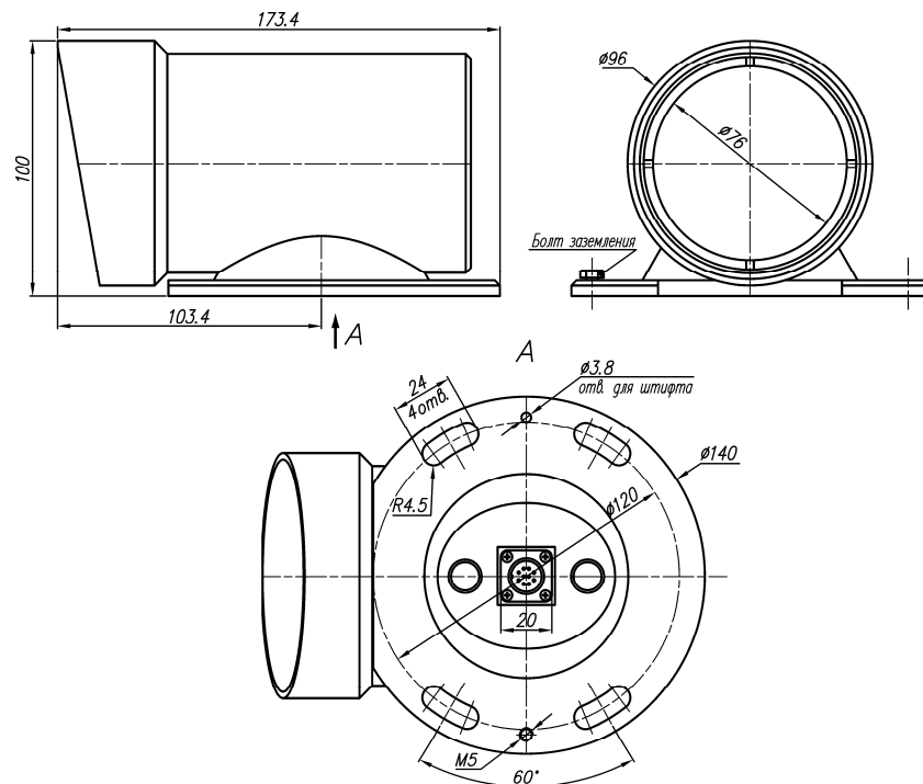
Рис. 2 Габаритно-установочные размеры.
